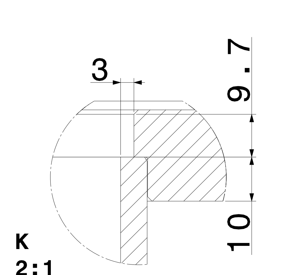
Flange CF-150
