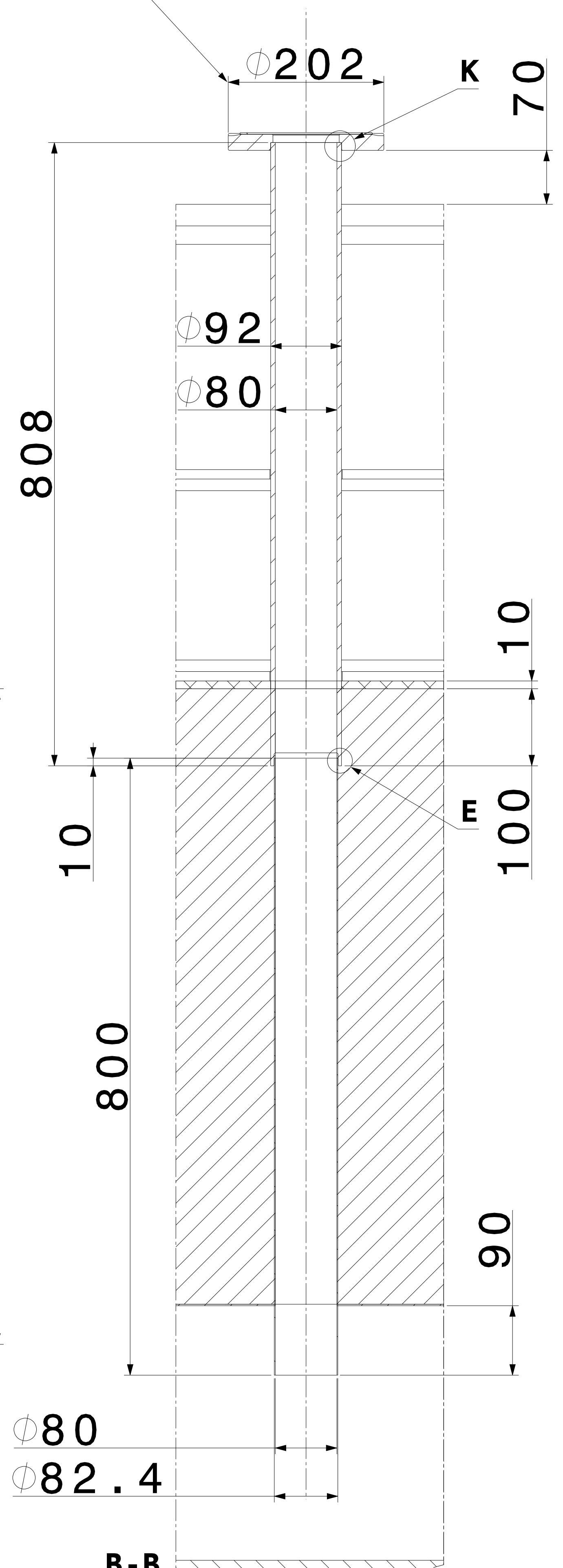
Flange CF-150
