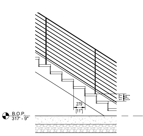
3 TREAD HEIGHT // DEPTH 1:25
