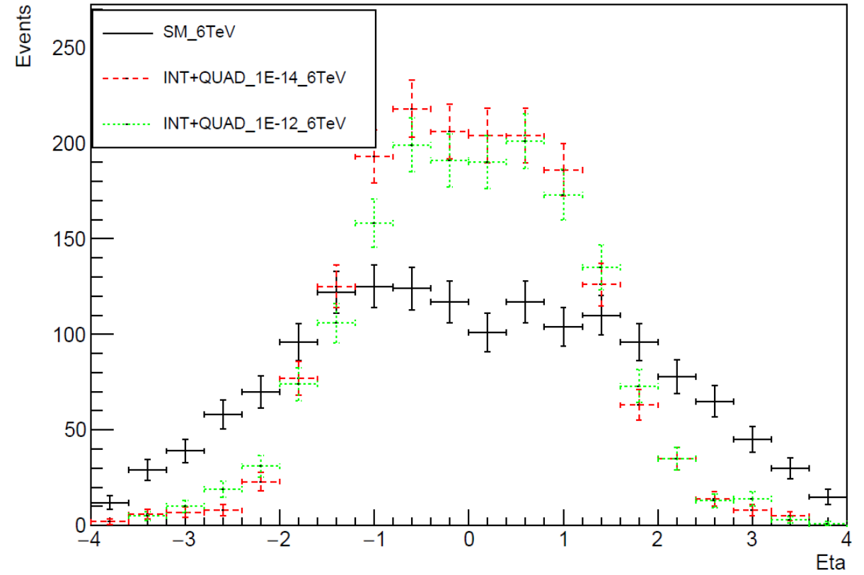
Muon
