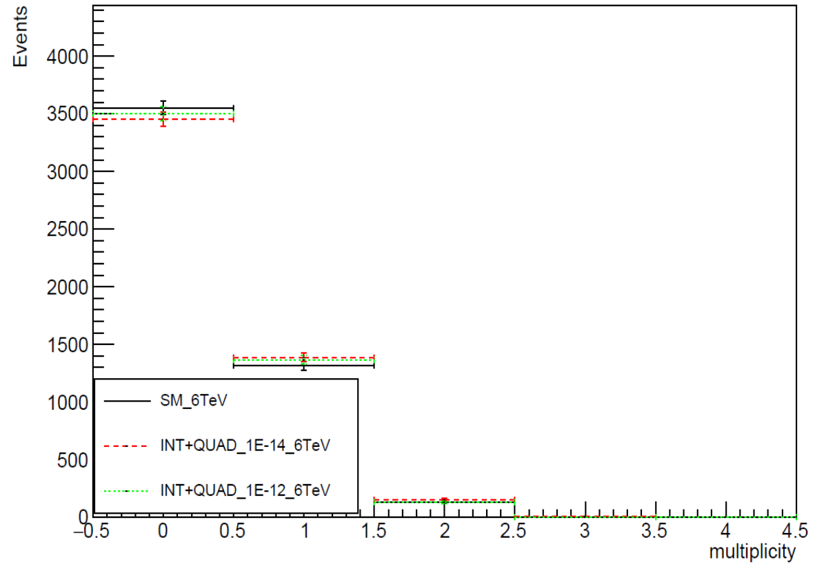
Muon
