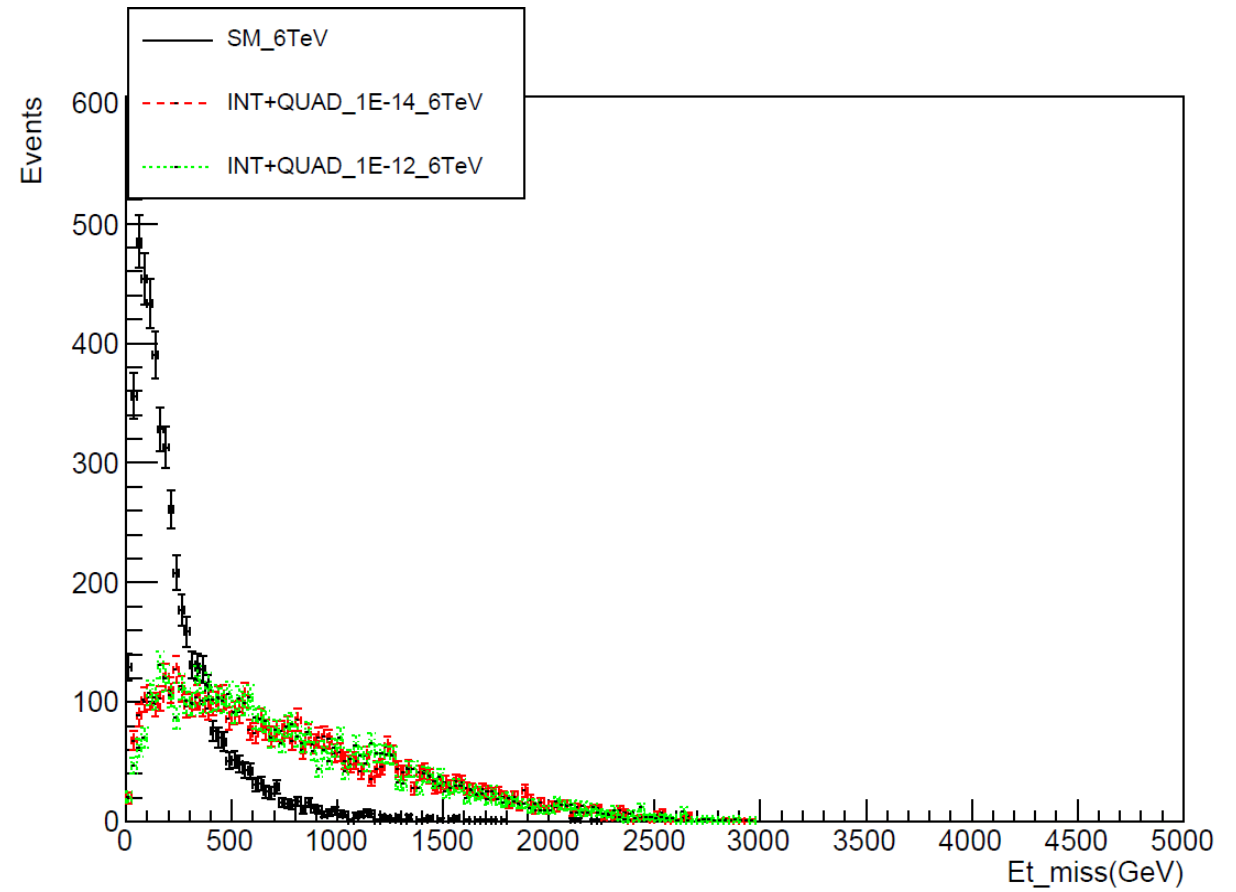
Missing Et
