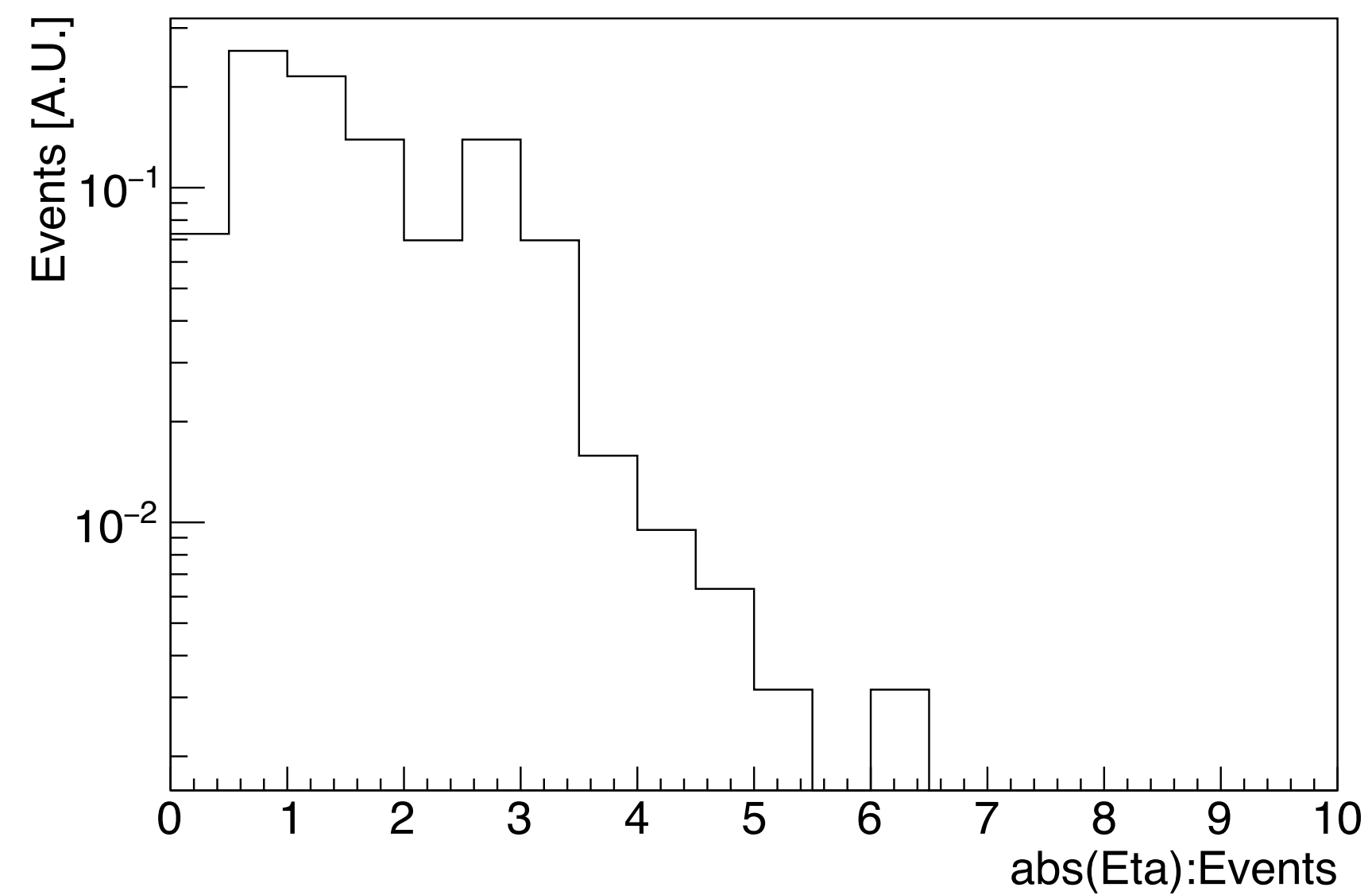
Eta distribution of W-daughters for WW->4q
