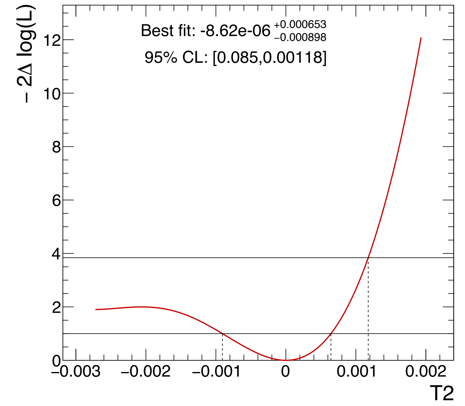
10 TeV T2
