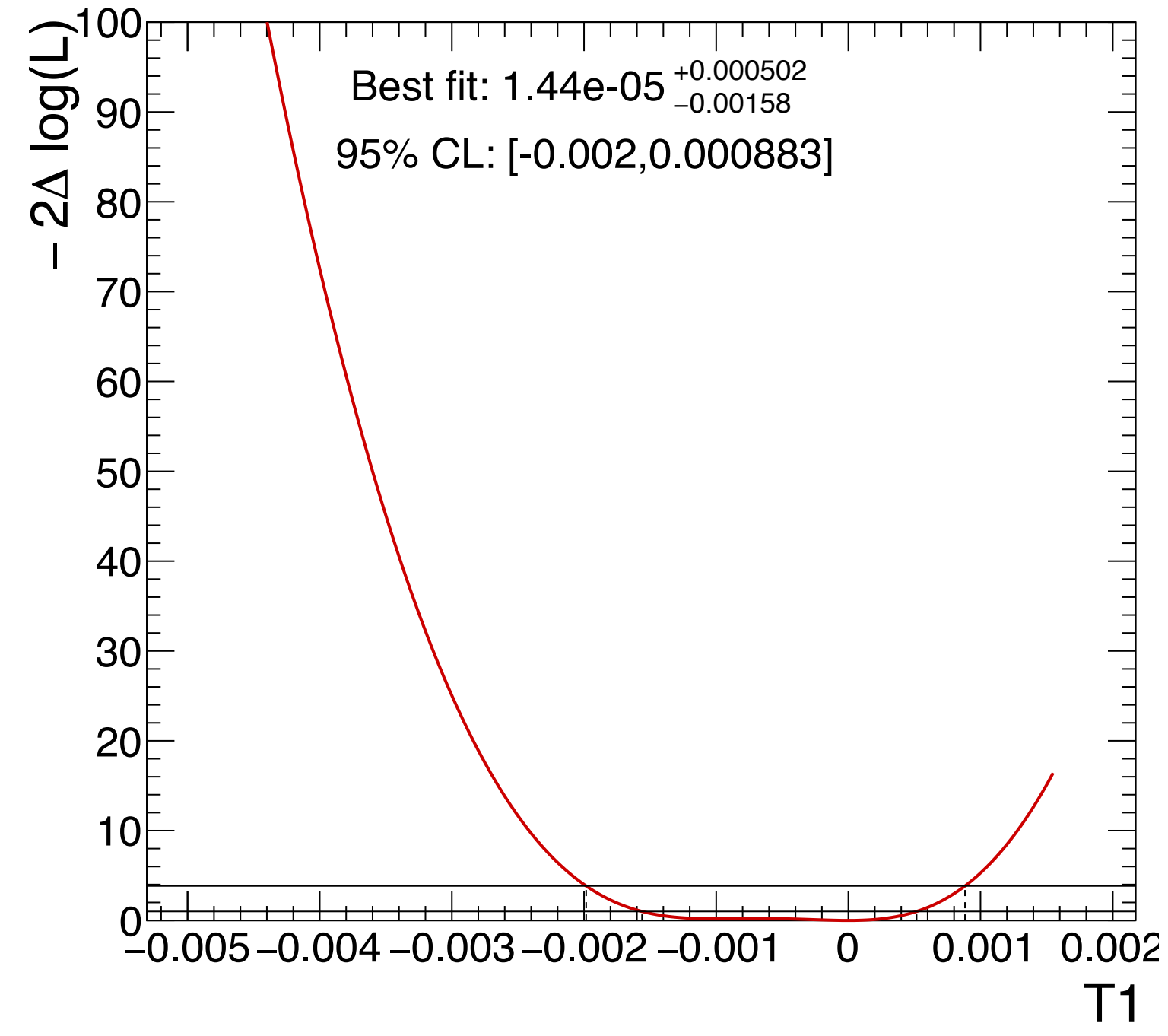
10 TeV T1
