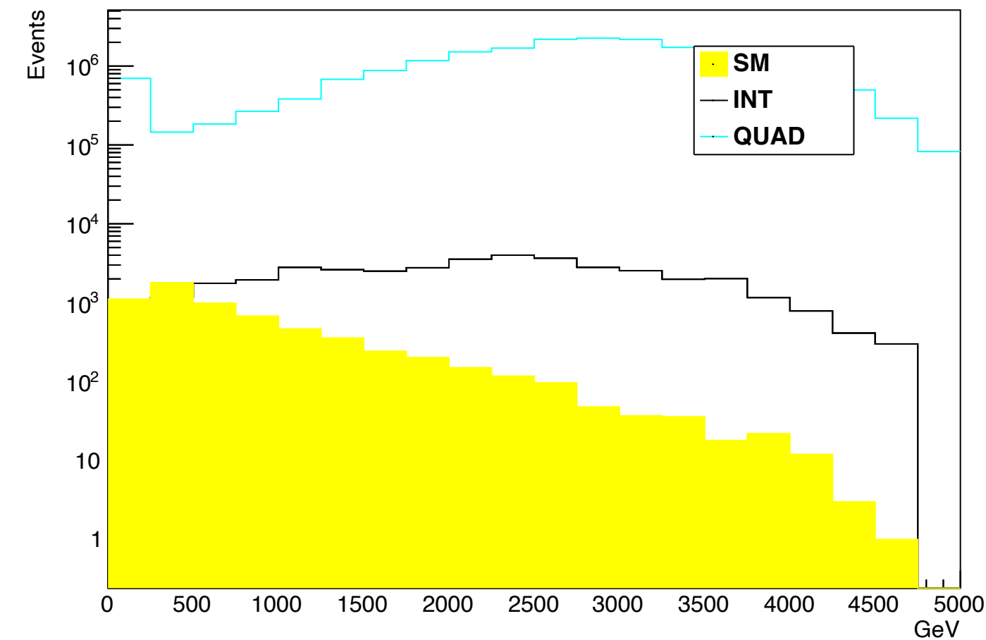
R_j_pT
