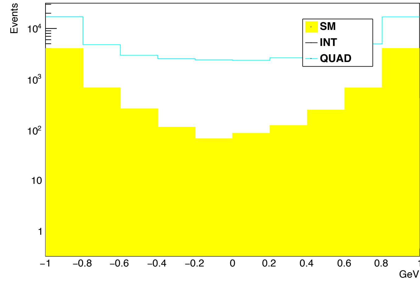
R_mu_cos
