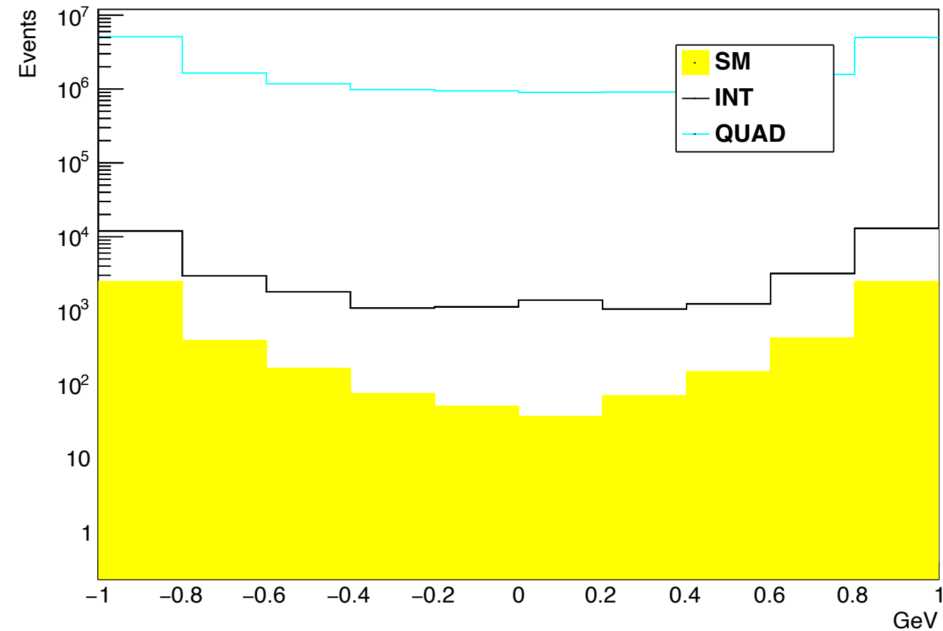
R_mu_cos
