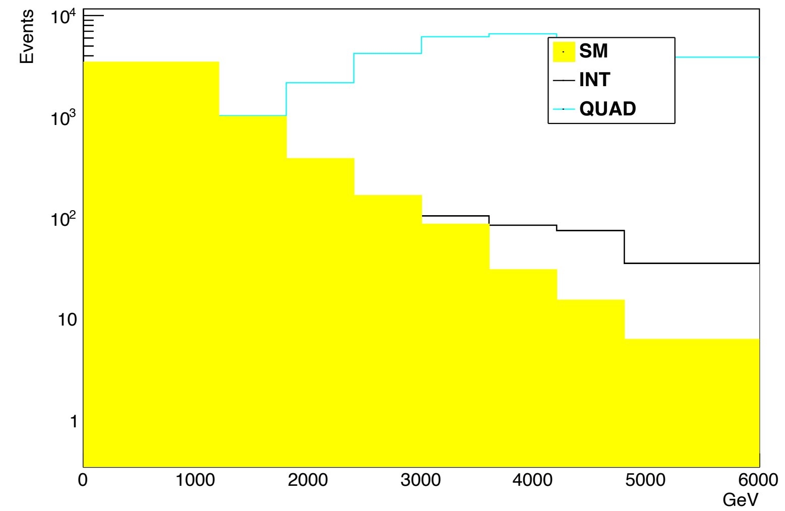
R_dijet_mass
