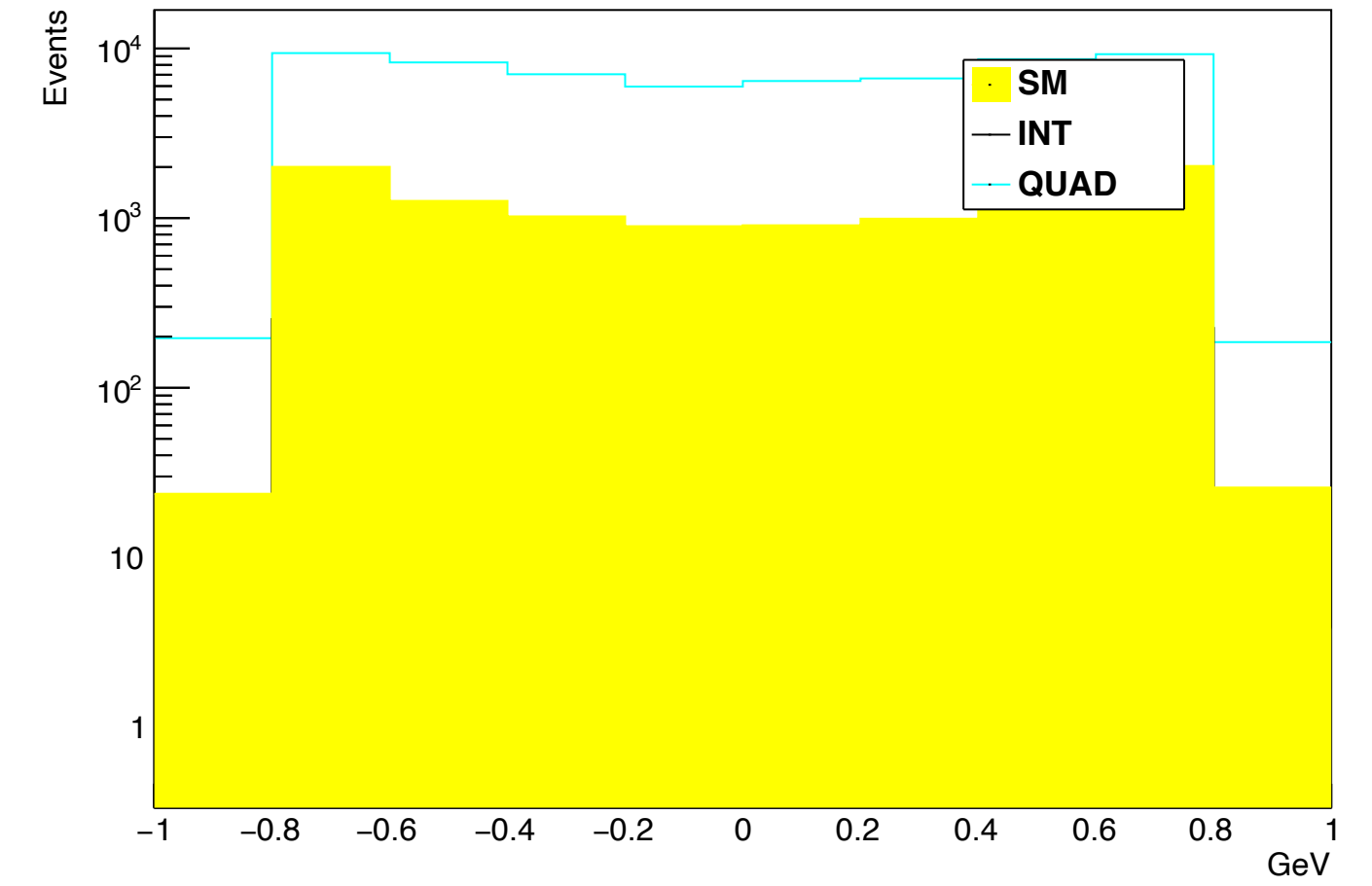
R_j_cos
