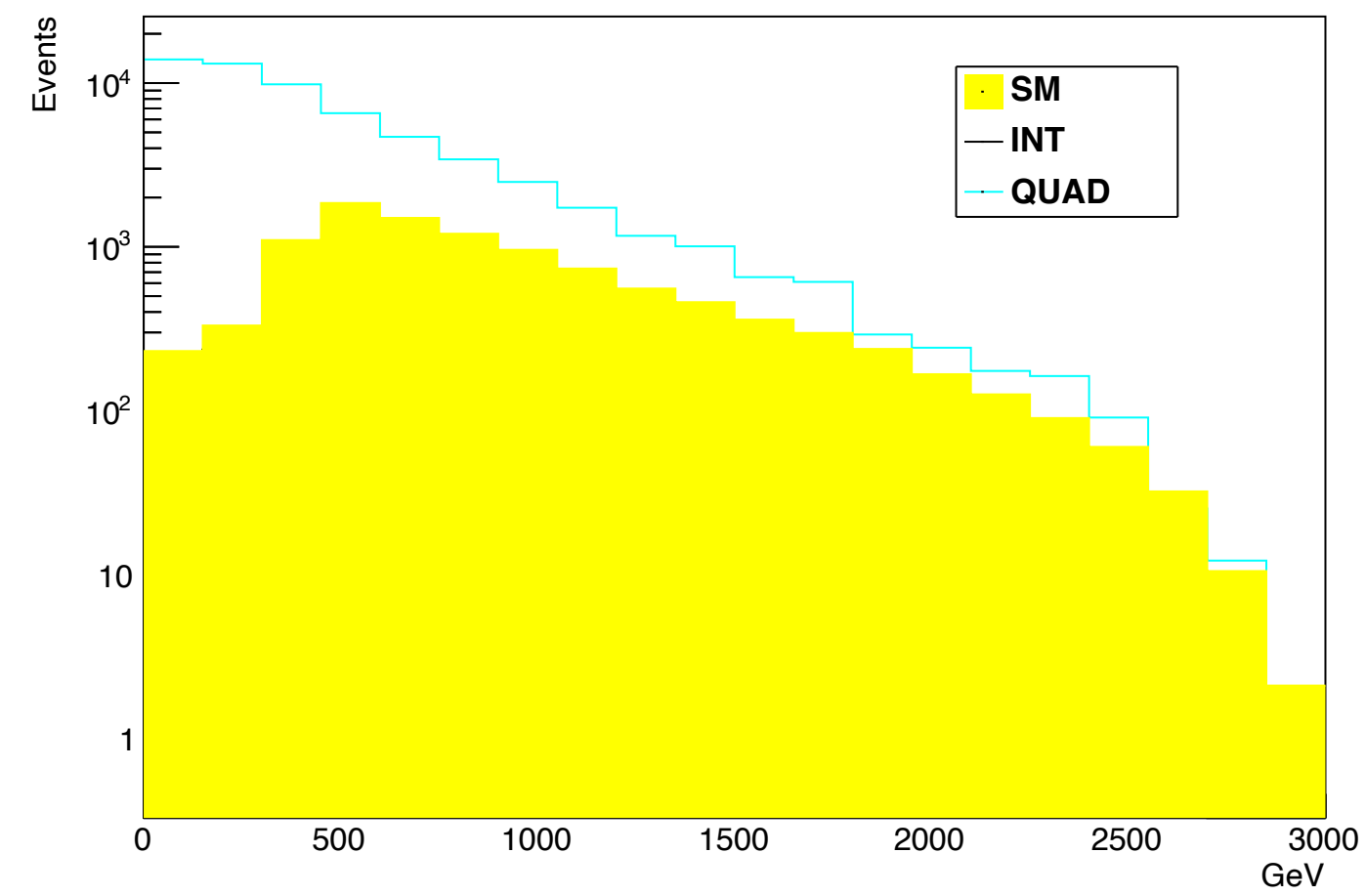
R_mu_pT
