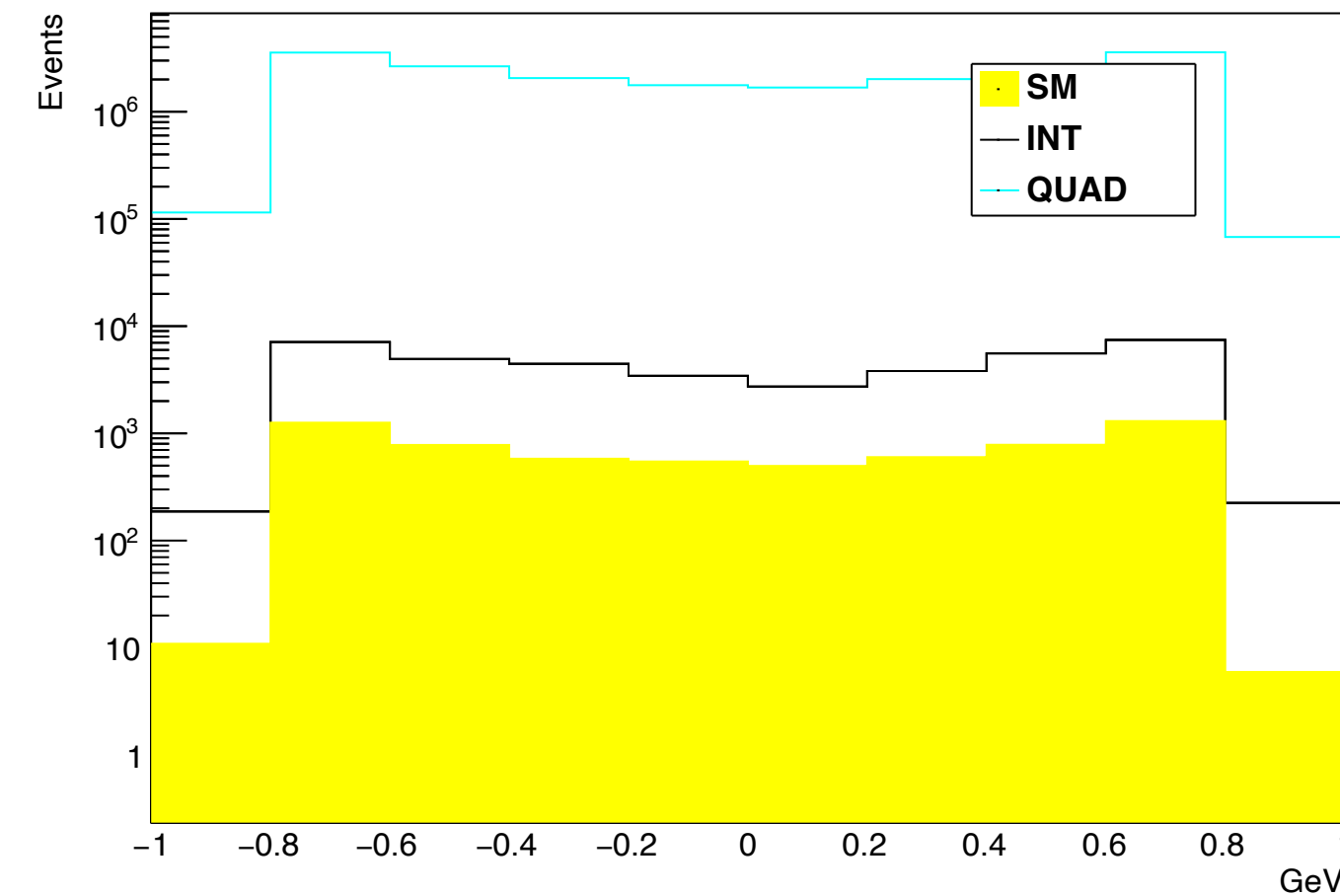
R_j_cos
