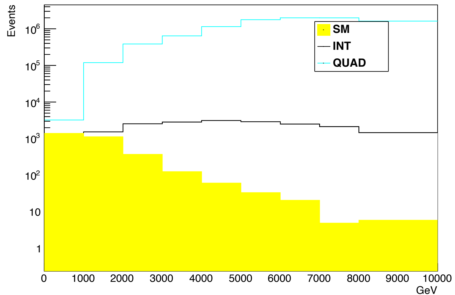
R_dijet_mass
