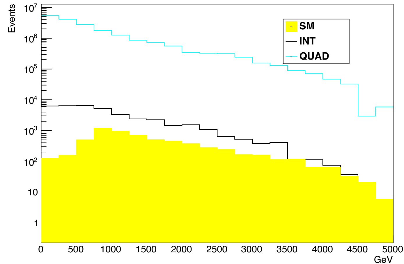
R_mu_pT
