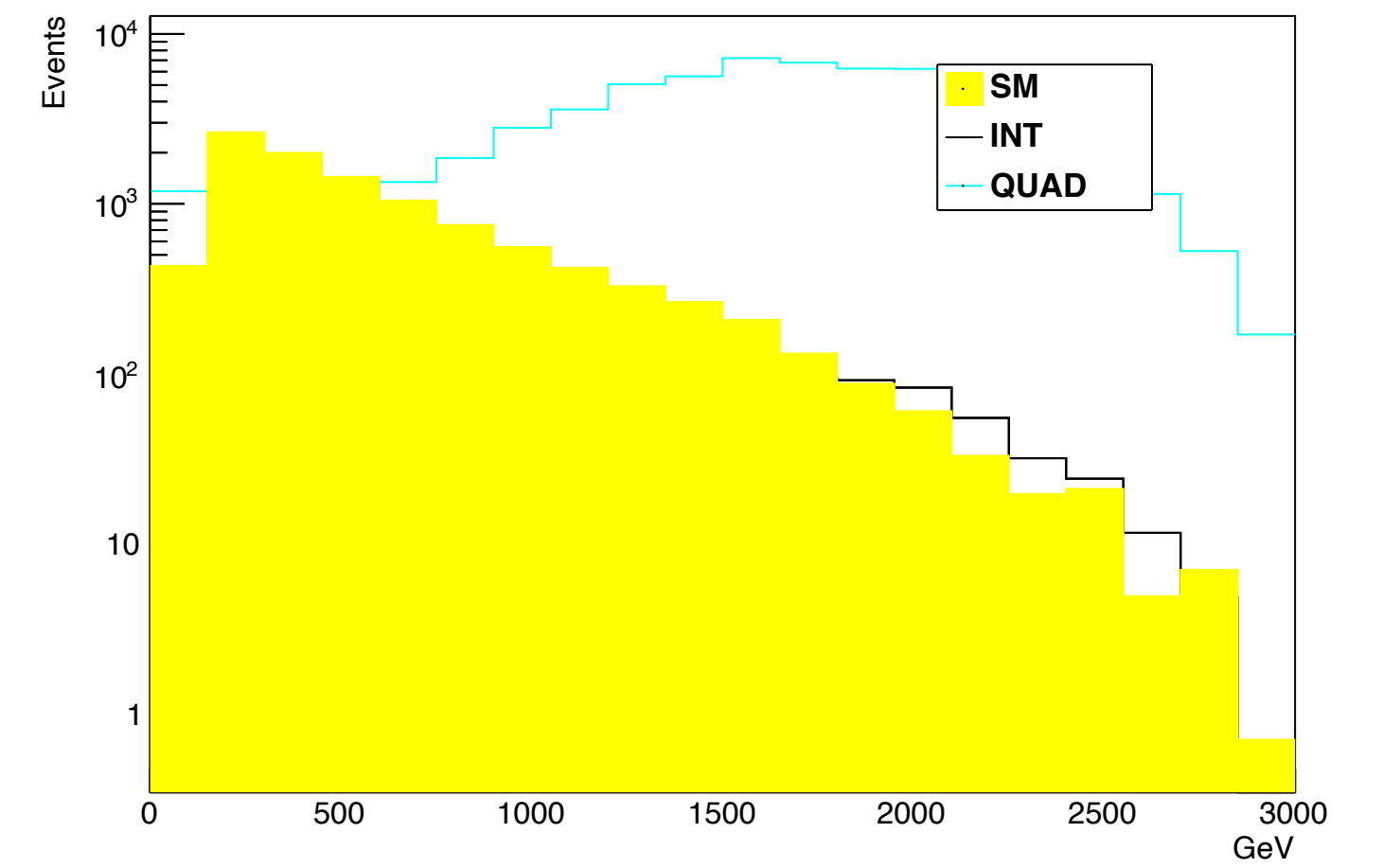
R_j_pT
