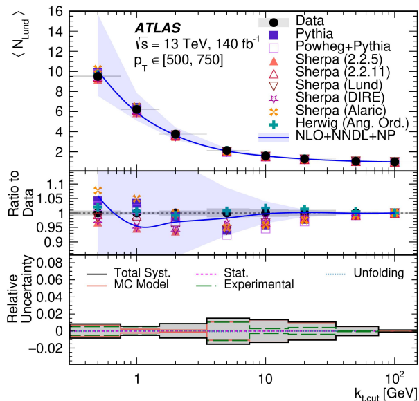
[ATLAS] arXiv:2402.13052
